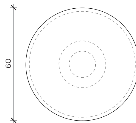
PIANTA | PLAN
